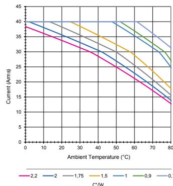
GNA - 40 A
